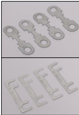
Schmelzstreifen Sicherung (U and O Type) (product codes: S3XXX, S4XXX-A and S4XXX-B)
