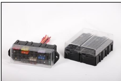
Modüler Güç Dağıtım ve Sigorta Kutusu (Ürün Kodu: FH1004)
